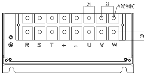
图 3-10 三相 55kW 主回路端子分布图
