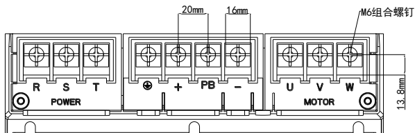
图 3-8 三相 30-37kW 主回路端子分布图
