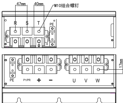
图 3-13 三相 110-132kW 主回路端子分布图
