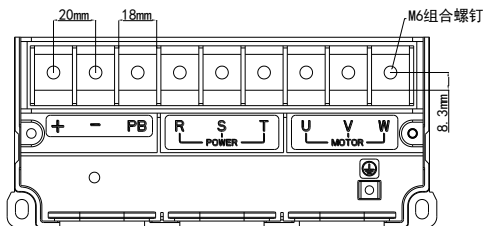
图 3-7 三相 15-22kW 主回路端子分布图
