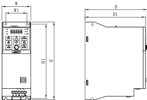
图 1-4 塑壳安装尺寸
