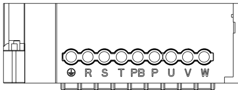
图 3-6 三相 7.5-11kW 主回路端子分布图
