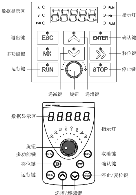
图 4-1 键盘示意图
