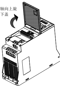
图 2-2 下盖板拆卸
