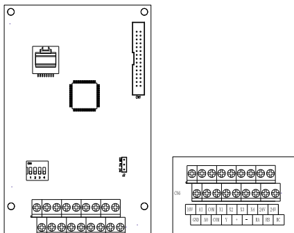
图 3-16 55-75kW 控制回路端子分布图
