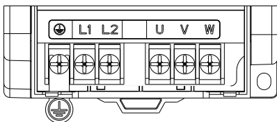
图 3-4 单相 0.75-2.2kW 主回路端子分布图
