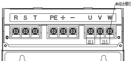
图 3-9 三相 45kW 主回路端子分布图
