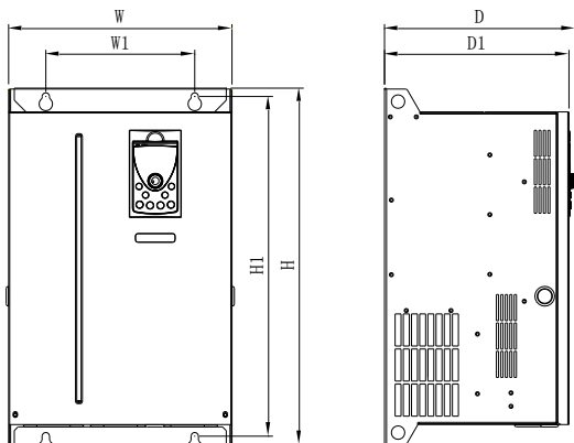
图 1-5 钣金安装尺寸
