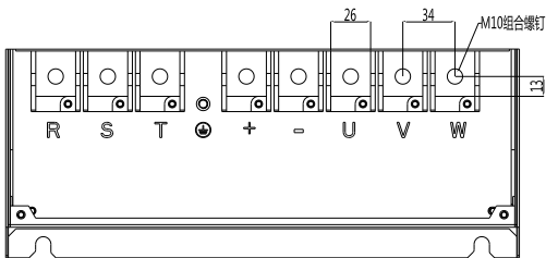
图 3-11 三相 75kW 主回路端子分布图
