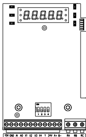
图 3-14 4.0-11kW 控制回路端子分布图
