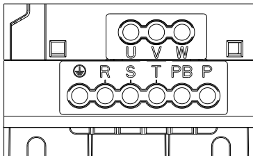
图 3-5 三相 0.75-5.5kW 主回路端子分布图
