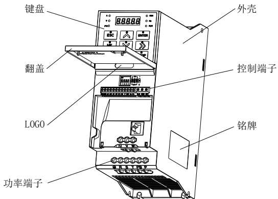
图 1-3 外壳机型各部分名称
