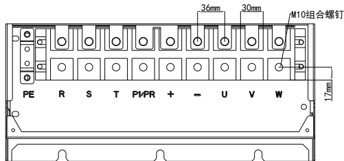
图 3-12 三相 90kW 主回路端子分布图
