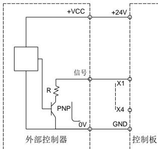
图 3-3 X 端子接线方式
